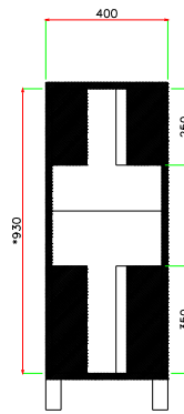
截面 A-A
